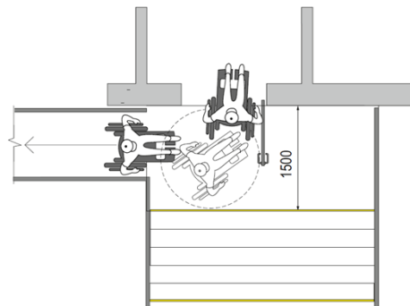
Рисунок 1.22. Схема маневрування кріслом колісним на ґанку
