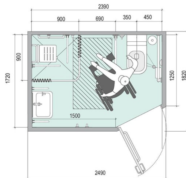
Рисунок 3.21. Приклад типового санітарно- гігієнічного приміщення. Тип 2
