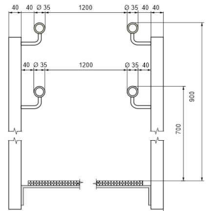
Рисунок 1.17. схема розрізу пандуса
