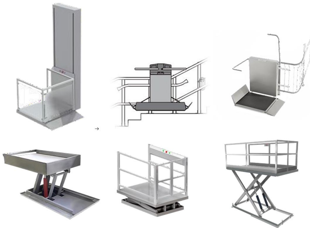
Рисунок 1.26. Типи підймальних пристроїв для облаштування танків
