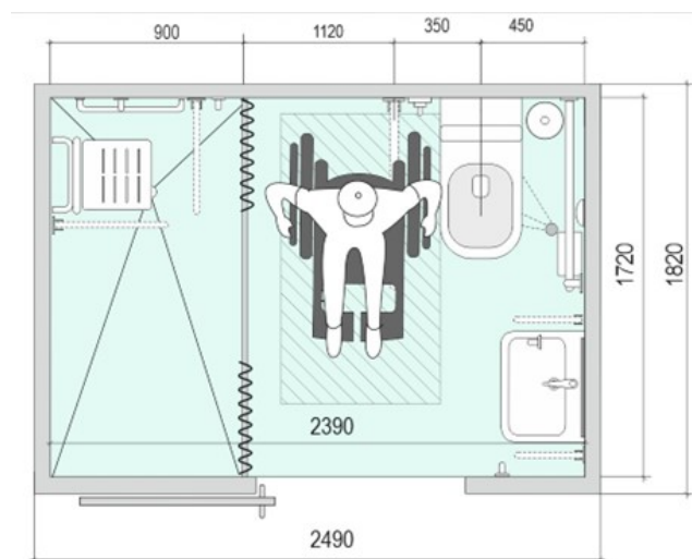
Рисунок 3.20. Приклад типового санітарно- гігієнічного приміщення. Тип 1
