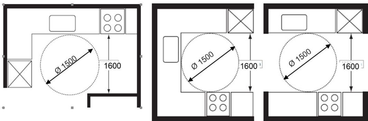
Рисунок 3.14. Варіанти розміщення обладнання в робочий кухні
