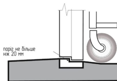
Рисунок 1.9. Поріг вхідного вузла
