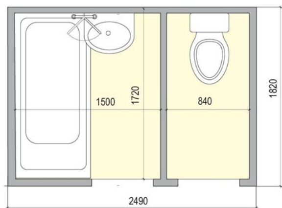
Рисунок 3.20. Приклад типового санітарно- гігієнічного приміщення. Тип 1
