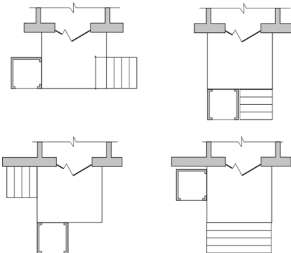
Рисунок 1.27. Взаємне розміщення підймальних пристроїв і сходів
