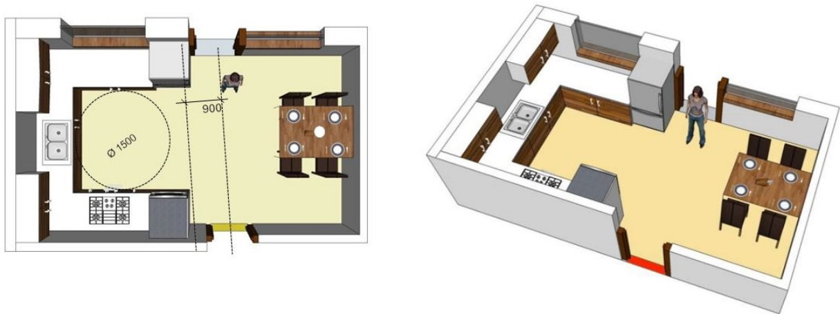
Рисунок 3.11. Схема умеблювання кухні-їдальні
