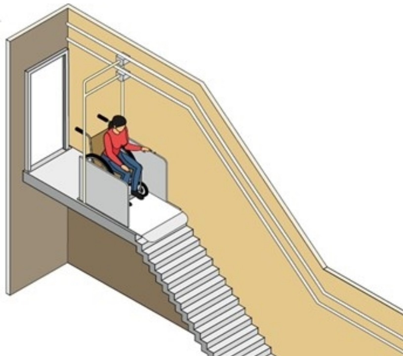
Рисунок 2.3. Схема влаштування похилого підймального пристрою на підвісах
