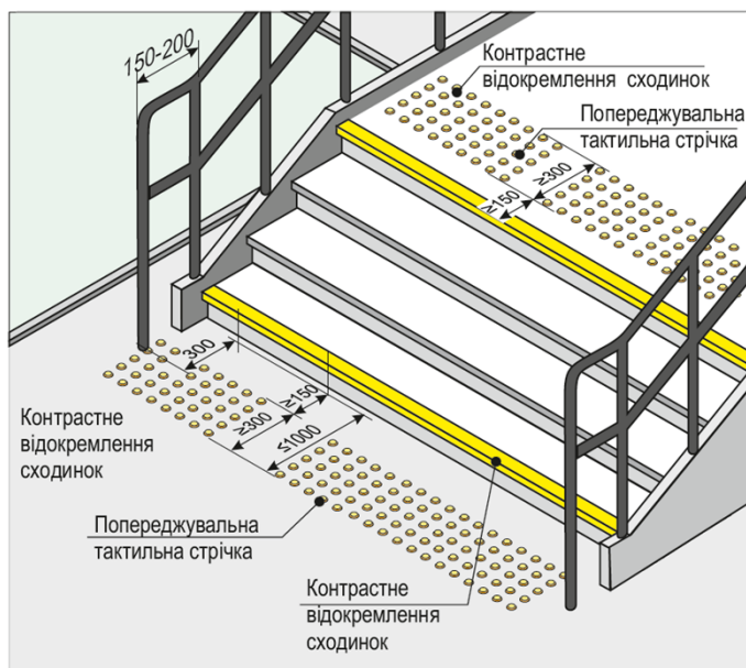
Рисунок 1.14. Облаштування сходинок
